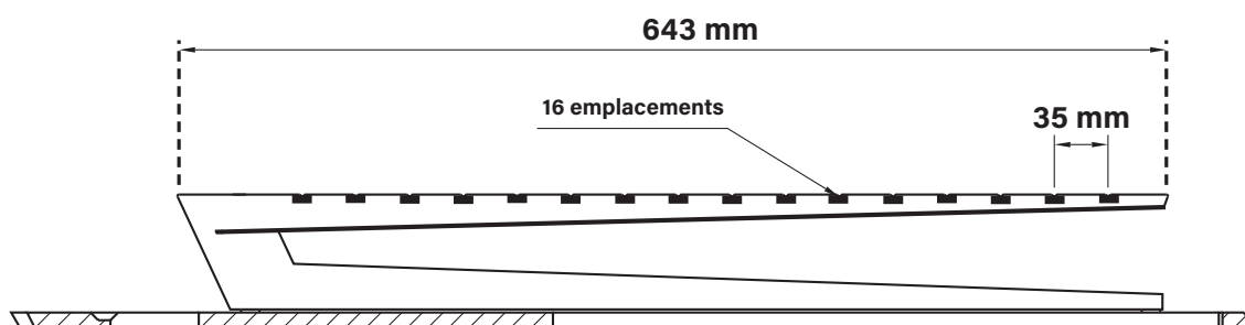
VUE DE DROITE
